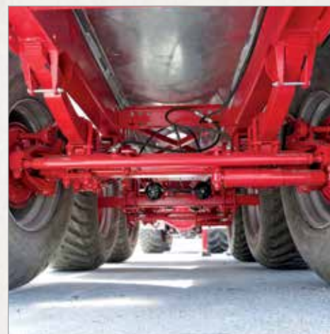
Tridem vzmeteno podvozje z listnatimi vzmetmi
